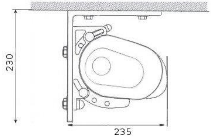
Encombrement plafond
