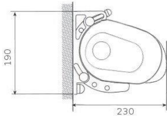
Encombrement face
