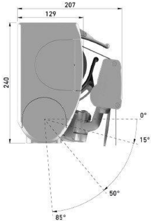
Encombrement bras standard
